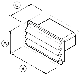
5 Outlet Grille, 222x89
