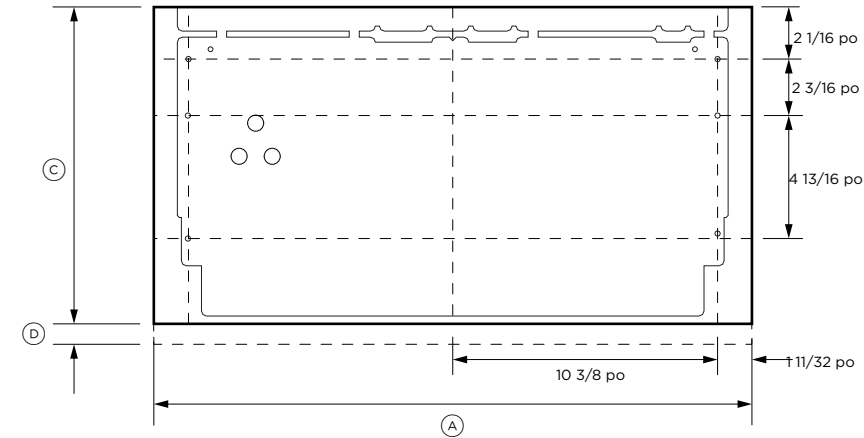
PANNEAU INFÉRIEUR - VUE ARRIÈRE
