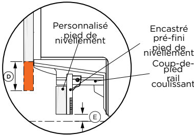
VUE EN COUPE DÉTAILLÉE 1 PROFONDEURS DE COUP-DE-PIED 2 3/26 - 4 3/4 PO
