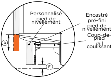
VUE EN COUPE DÉTAILLÉE 1 PROFONDEURS DE COUP-DE-PIED 1 9/16 - 4 3/4 PO
