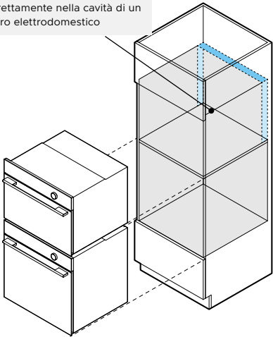
Opzioni per la superficie minima totale di ventilazione
