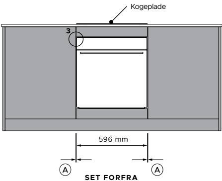
SET FORFRA
