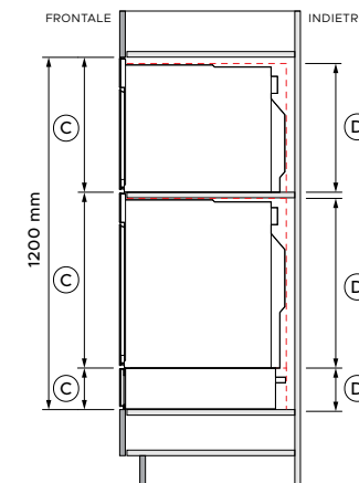
ESEMPIO VISTA PROFILO
