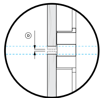
DETALLE 2 VISTA LATERAL
