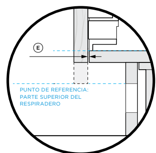
DETALLE 3 VISTA LATERAL
