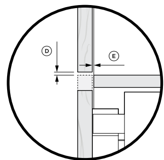
DETALLE 1 VISTA LATERAL
