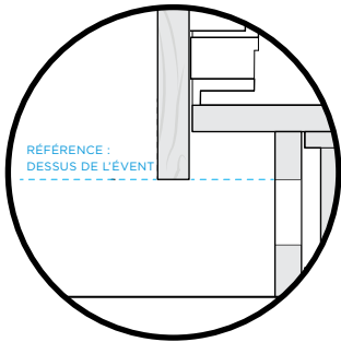
DÉTAIL A LA BASE DE LA PORTE DOIT ÊTRE ALIGNÉE SUR LE HAUT DE L'ÉVENT OU AU-DESSUS DE CELUI-CI
