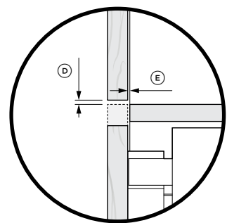
DÉTAIL 1 VUE LATÉRALE
