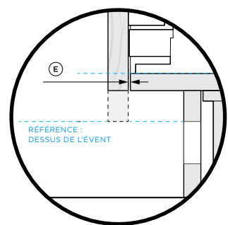
DÉTAIL 3 VUE LATÉRALE
