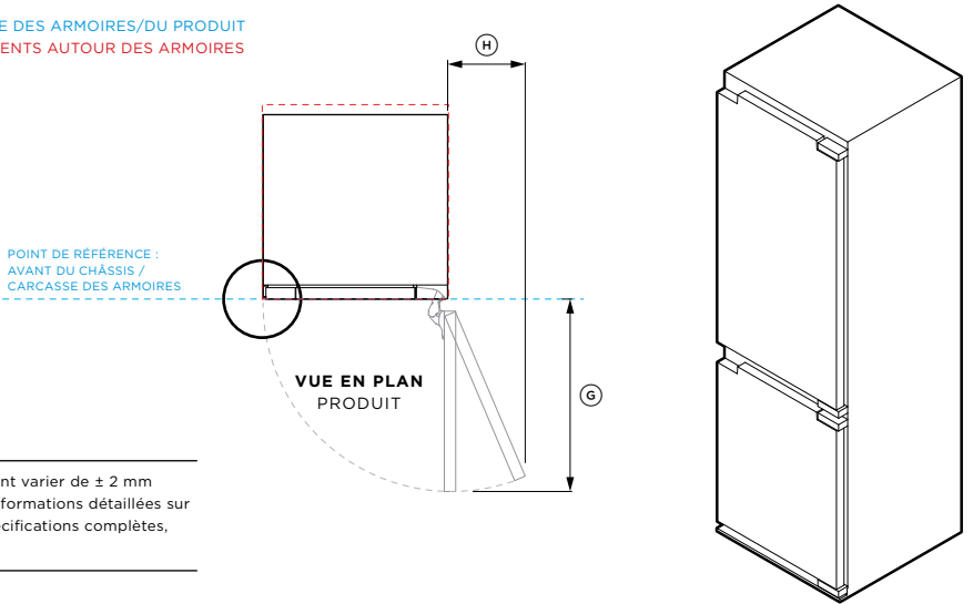
VUE EN PLAN DÉTAILLÉE PRODUIT AVEC ARMOIRES
