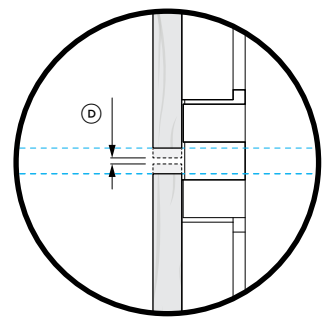
DÉTAIL 2 VUE LATÉRALE
