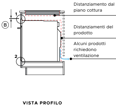
VISTA PROFILO
