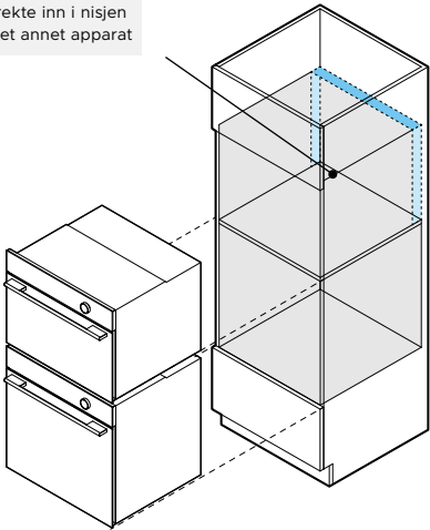
Alternativer for minimum ventilasjonsareal totalt
