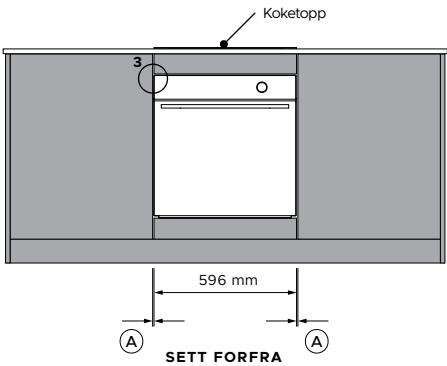
SETT FORFRA
