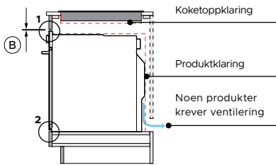
PROFILVISNING
