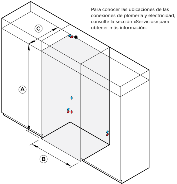
VISTA ISOMÉTRICA
