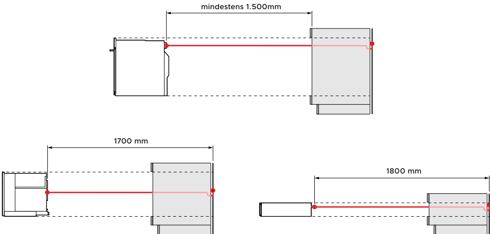
SEITENANSICHT
