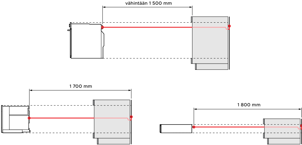
PROFIILINÄKYMÄ
