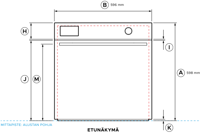
ETUNÄKYMÄ
