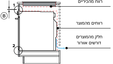
מבט מהצד
