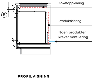
PROFILVISNING
