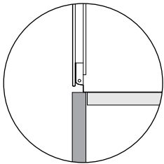
DETALJ 2 PROFILVISNING
