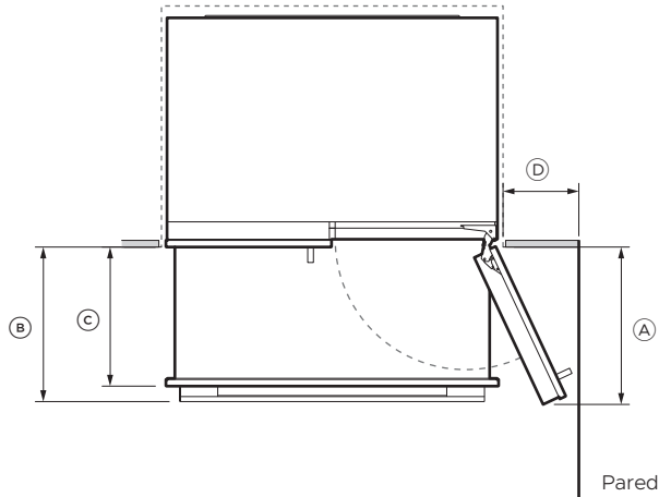
APERTURA DE PUERTA DE 115°
