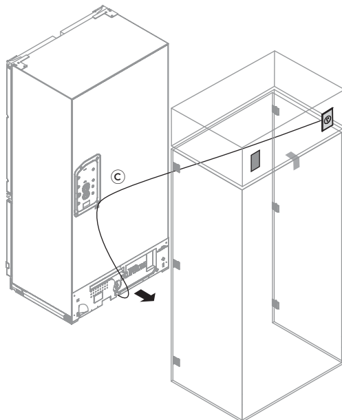
Conexión por encima de la cavidad
