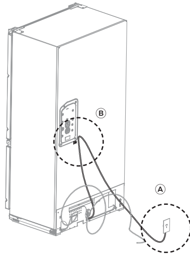
Conexión en la parte posterior de la cavidad
