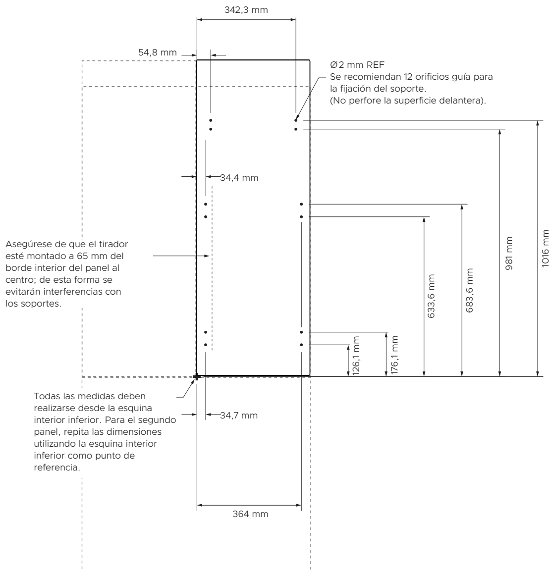
PANEL SUPERIOR – VISTA POSTERIOR
