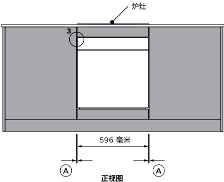
正视图
