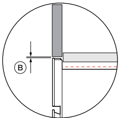
DETAIL 1 ZIJAANZICHT
