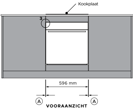
VOORAANZICHT
