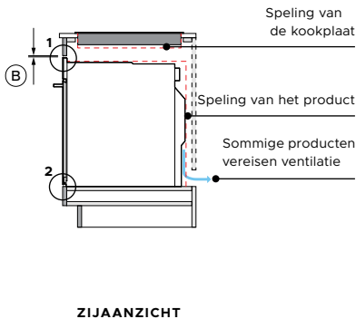
ZIJAANZICHT
