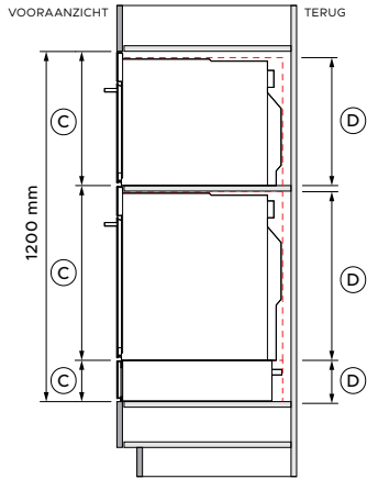
VOORBEELD ZIJAANZICHT
