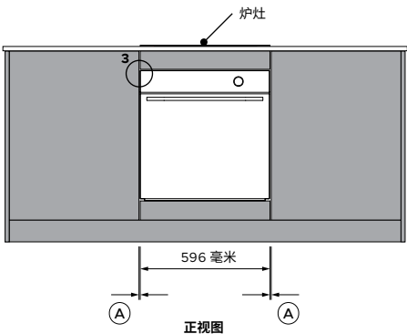
正视图
