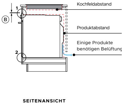
SEITENANSICHT
