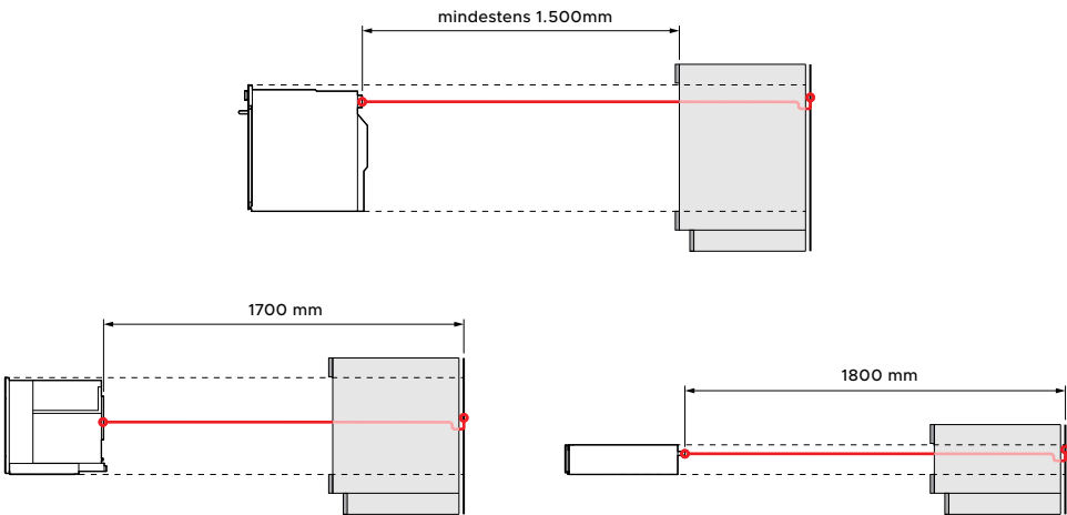
SEITENANSICHT
