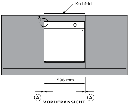
VORDERANSICHT
