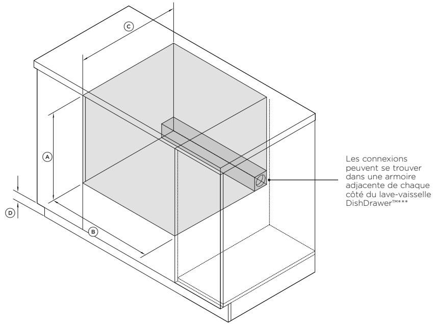
ISOMÉTRIQUE
