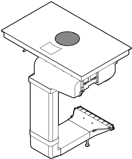
ISOMETRISCHE RÜCKANSICHT
