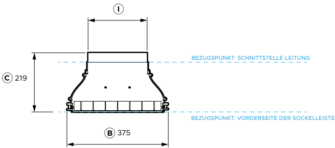
DRAUFSICHT
