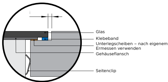
DETAIL B VORDERANSICHT Arbeitsplatte mit Kochfeld, flächenbündige Installation
