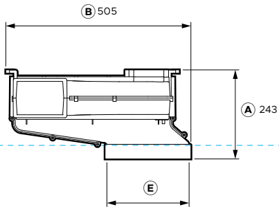
VORDERANSICHT
