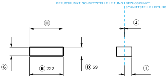
VORDERANSICHT
