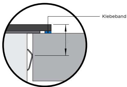
DETAIL – ERGÄNZUNG VORDERANSICHT Arbeitsplatte mit Kochfeld, aufliegende Installation
