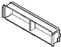
ISOMETRISCHE VORDERANSICHT 62MM-ERWEITERUNGSBLOCK
