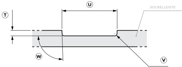
VORDERANSICHT SCHRANKAUSSCHNITT
