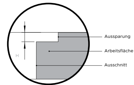
DETAIL A VORDERANSICHT – QUERSCHNITT Arbeitsplatte ohne Kochfeld, Aussparung für flächenbündige Installation
