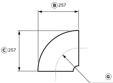
DRAUFSICHT
