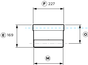
VORDERANSICHT
