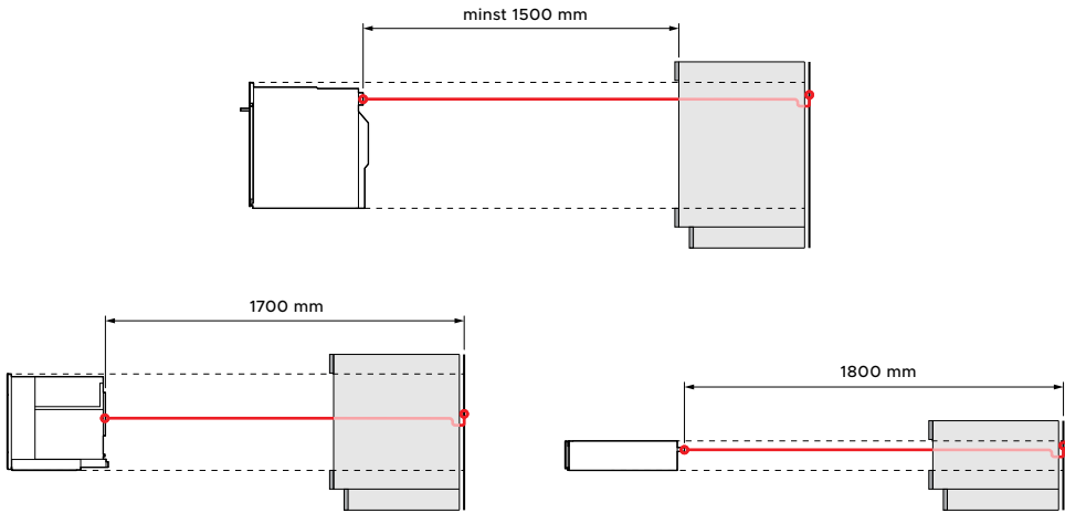
PROFILVY
