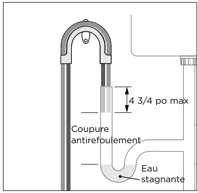
VUE DES DÉTAILS - INSTALLATION DU TUYAU VERTICAL
