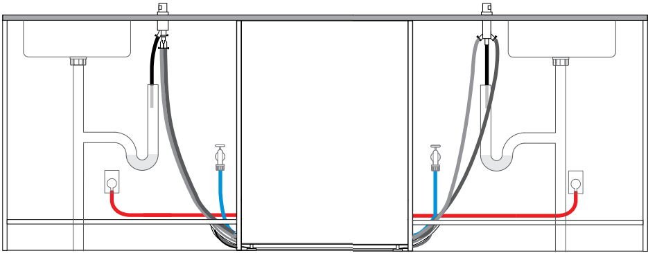
INSTALLATION DE LA COUPURE ANTI-RETOUR SIMPLE
