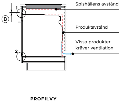
PROFILVY
