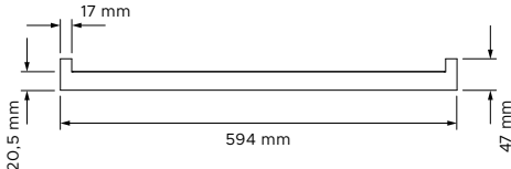
VOORAANZICHT
