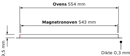
BOVENAANZICHT
