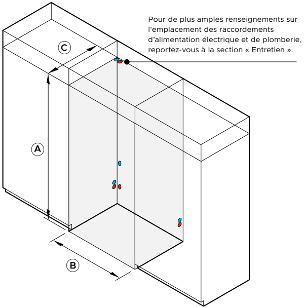
VUE ISOMÉTRIQUE
