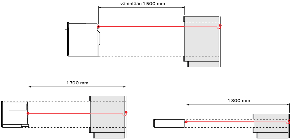
PROFIILINÄKYMÄ
