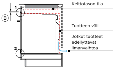
PROFIILINÄKYMÄ
