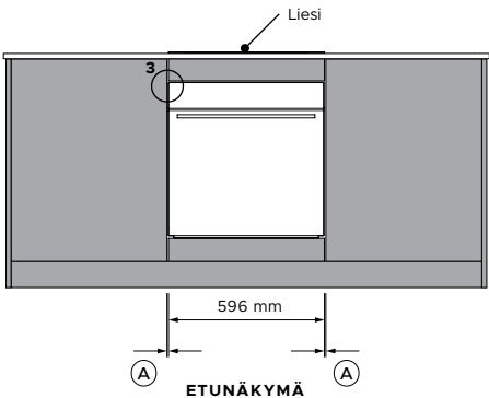
ETUNÄKYMÄ
