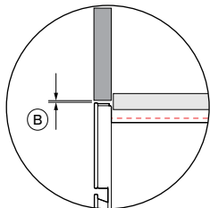
DETAIL 1 SEITENANSICHT
