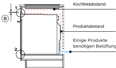
SEITENANSICHT
